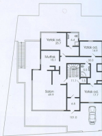
Zemin kat planı (S 285.3)
